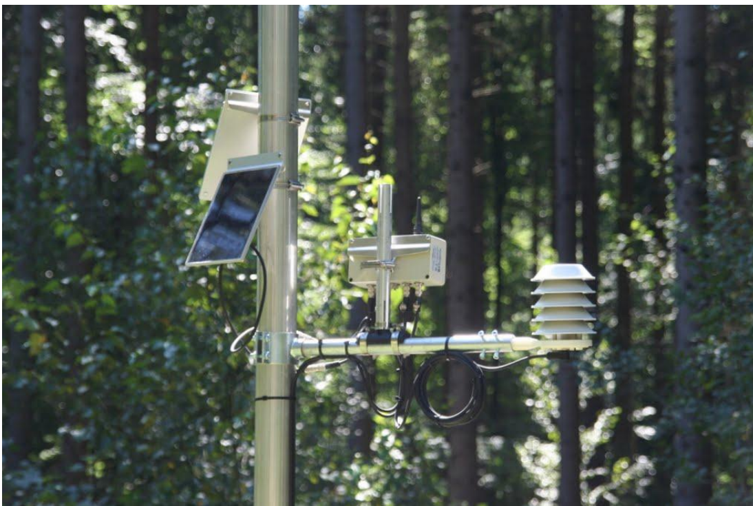
Solarpanel, GPRS-Sender und Vaisala-Sonde
